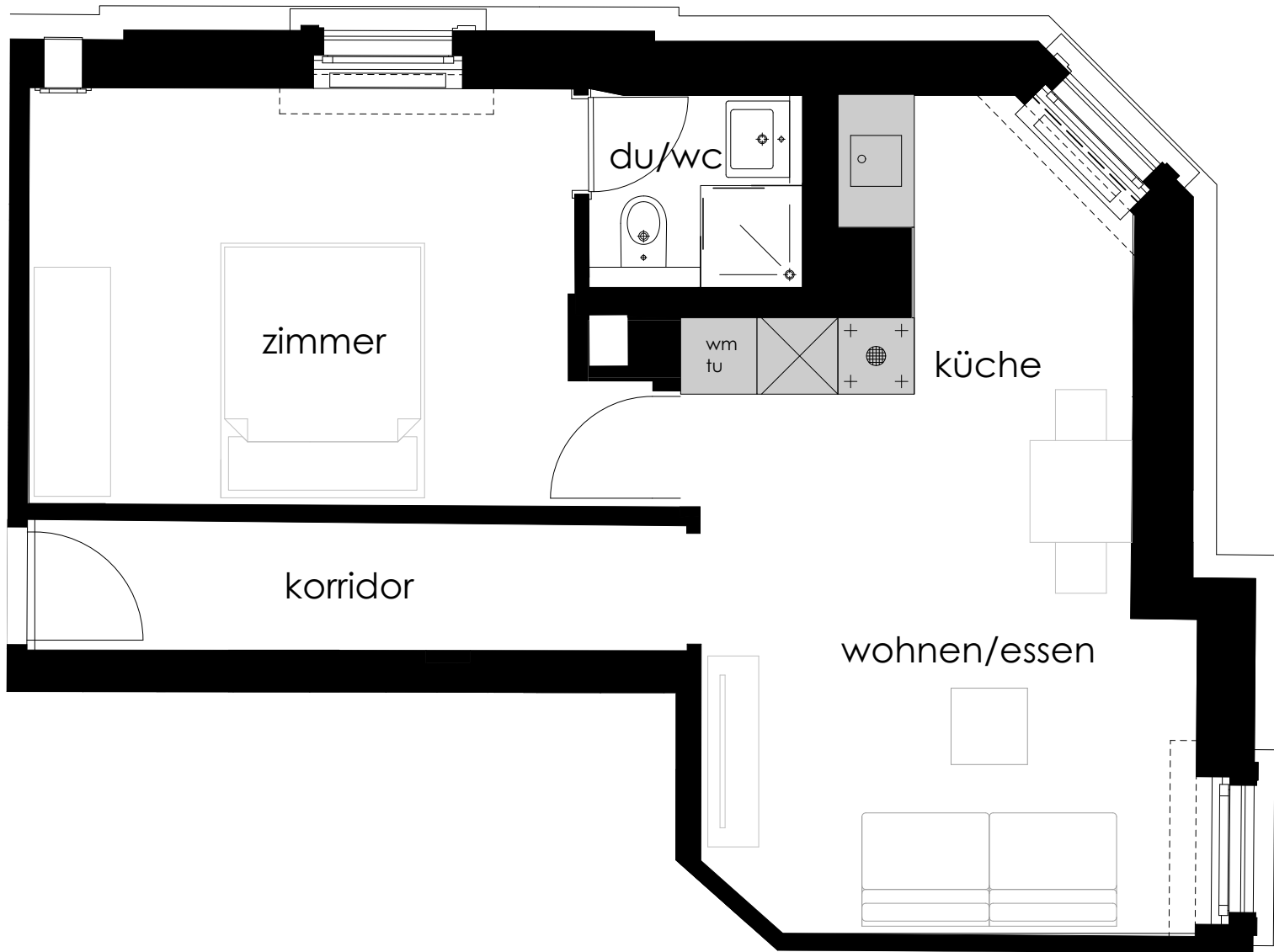
3.obergeschoss 1:50
