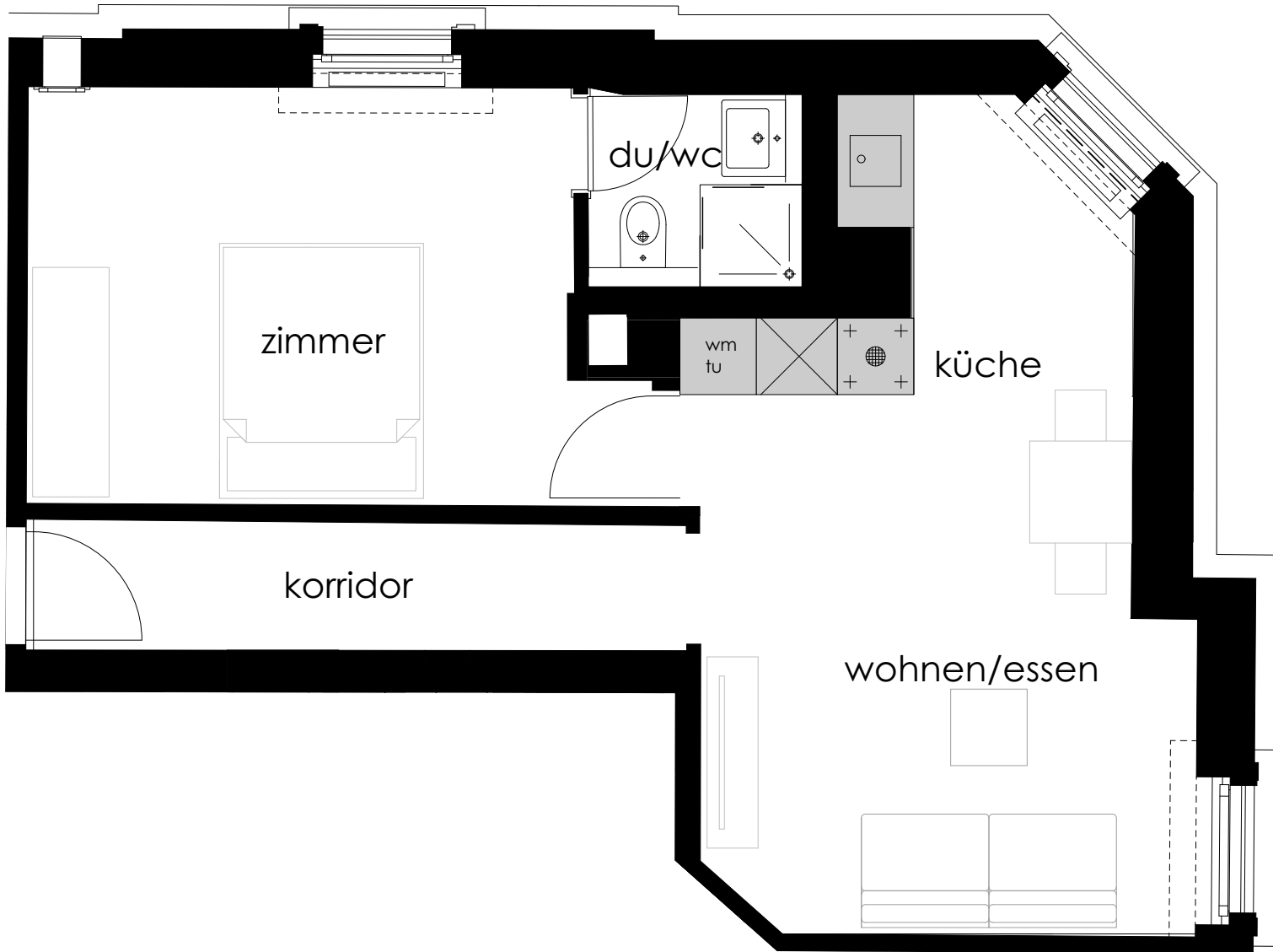
1.obergeschoss 1:50
