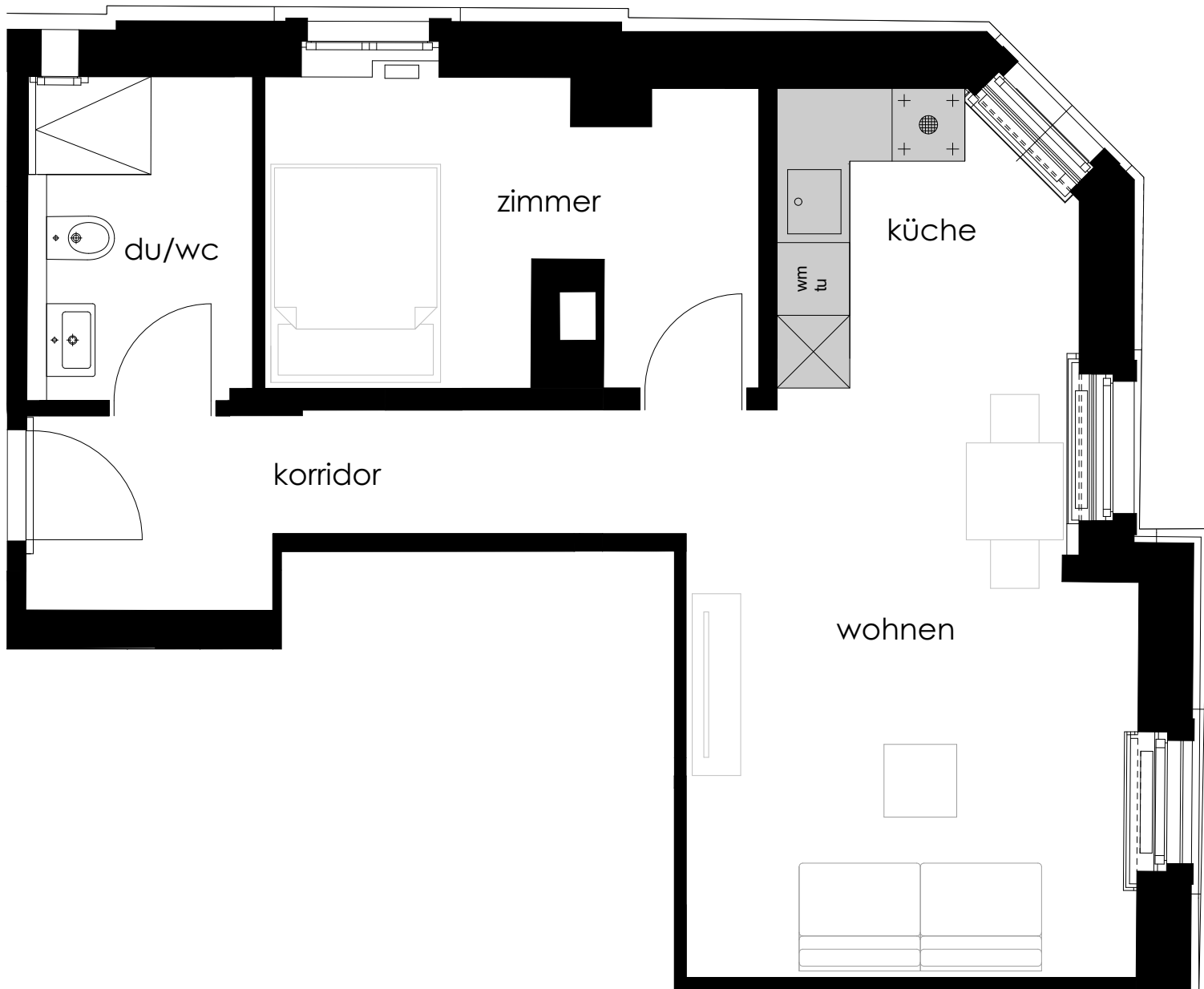
erdgeschoss 1:50
